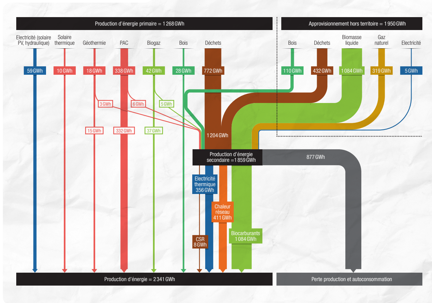
Schéma de la production d'énergie dans et hors du territoire (source : Agence Locale de l'Energie et du Climat de la métropole bordelaise et de la Gironde)
